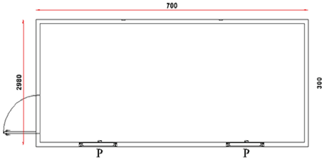
SK 103 PLAN
