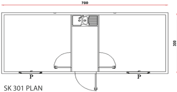
SK 301 PLAN
